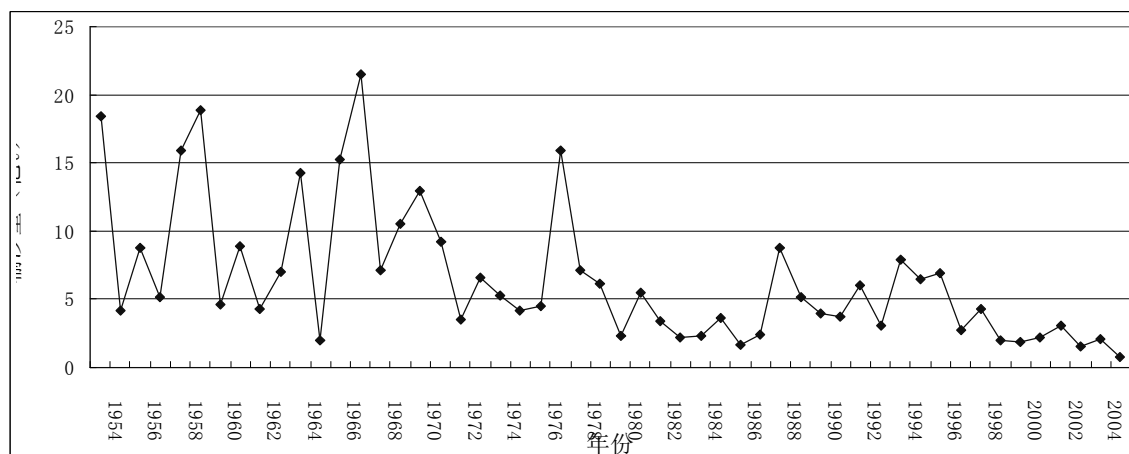
图2 1954—2005年河龙区间实测年输沙量
