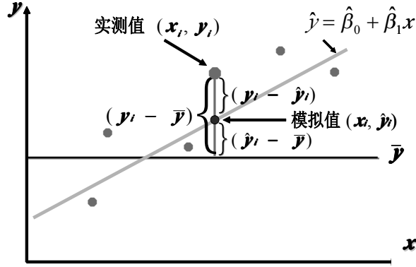
图6 回归分析原理示意
