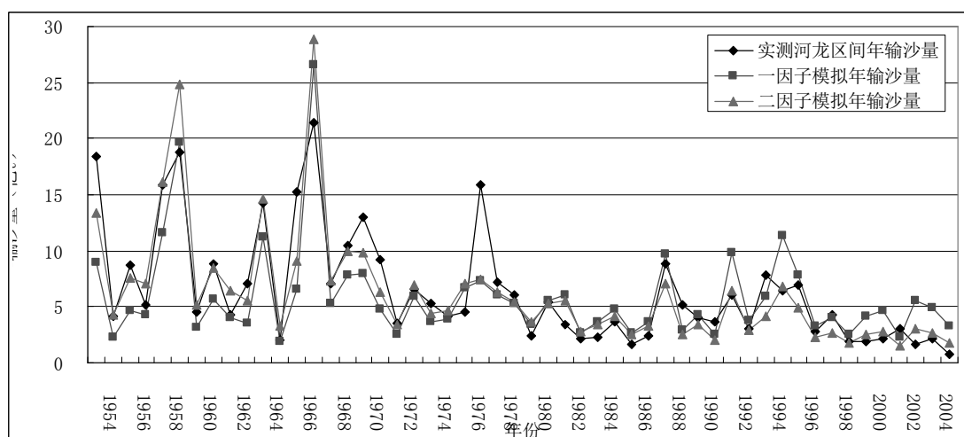
图5 1954—2005年不同因子模拟结果比较
