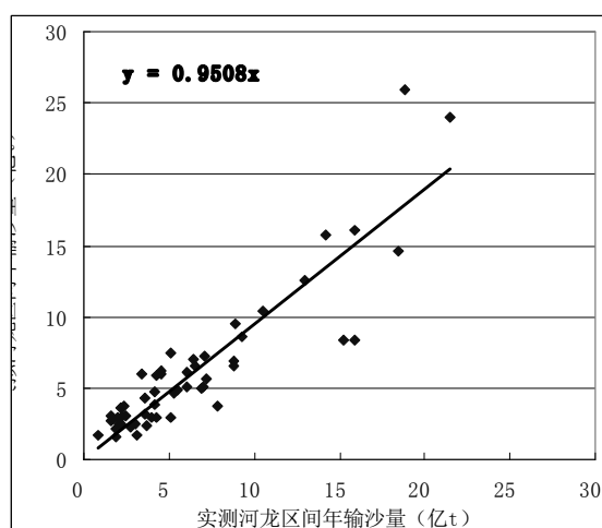
图4 1954—2005年实测年输沙量与模拟年输沙量的散点图
