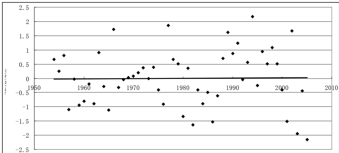
图 7 回归标准化残差散布
