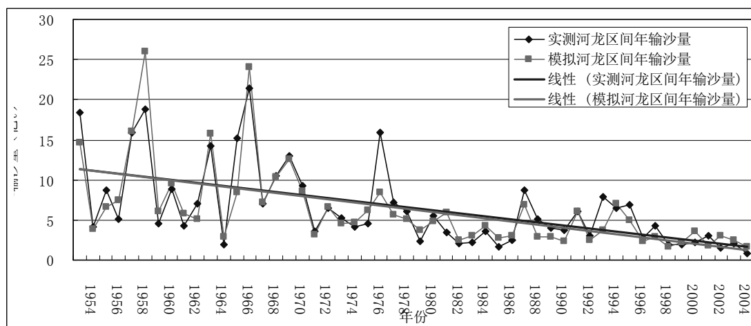
图3 1954—2005 年实测年输沙量与模拟年输沙量比较
